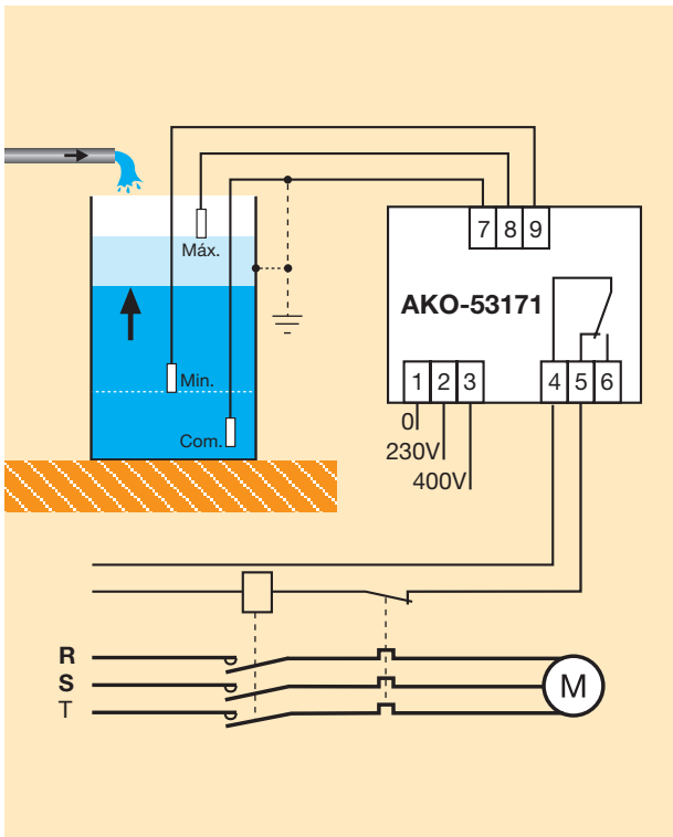
Llenado (depósito) Filling (tank)
